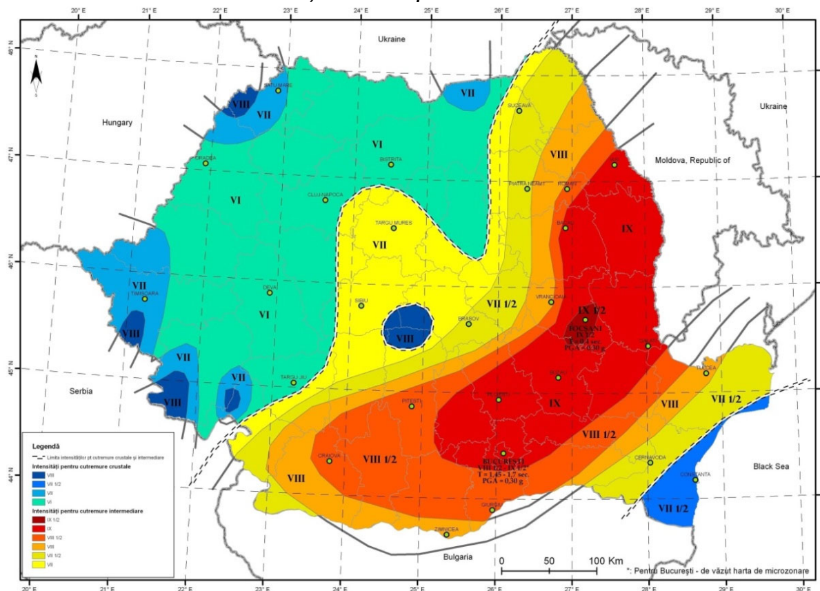
Harta intensitatii seismice, in situatia producerii cutremurului maxim credibil
